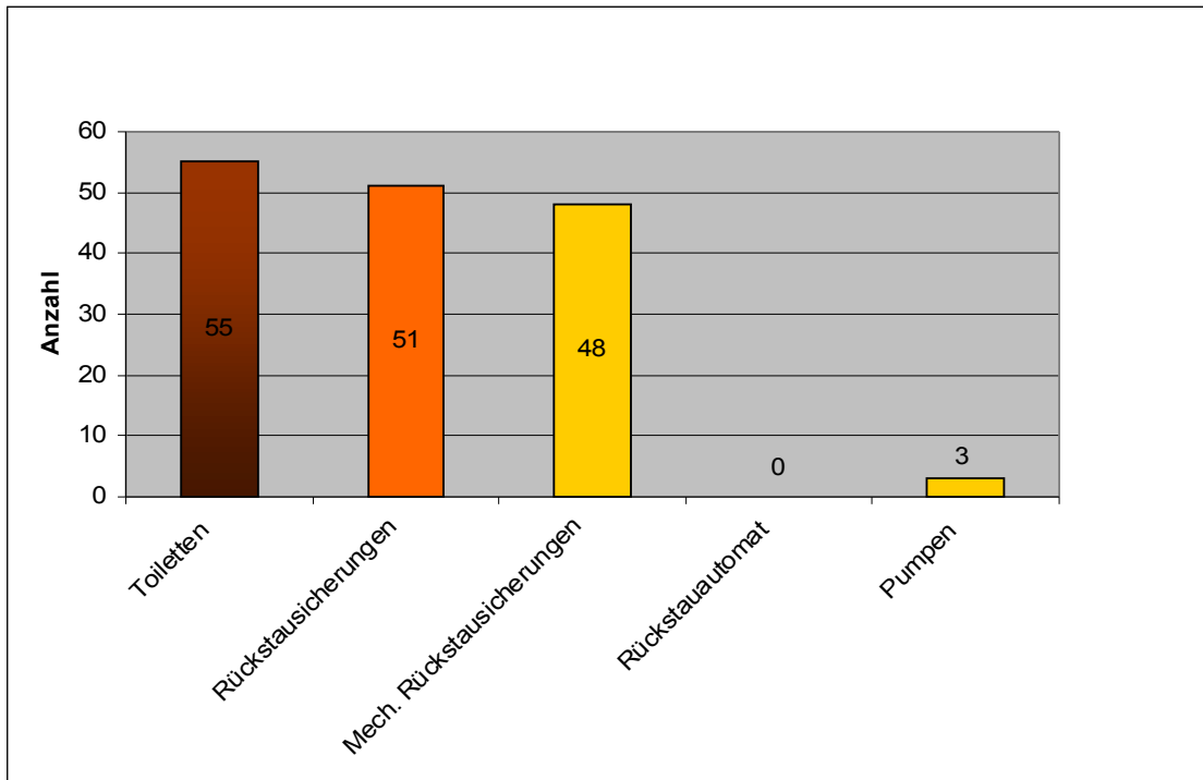
Abb. 3: Toiletten im Keller und verwendete Arten von Rückstausicherungen
